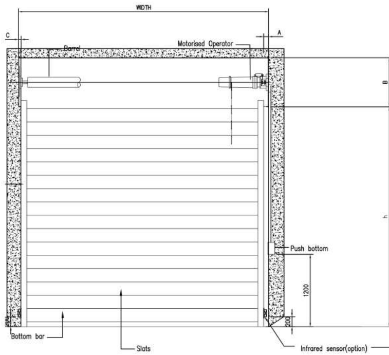
ELEVATION A
